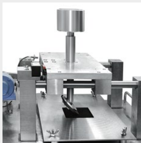
Устройство для проведения «испытания каблуком»
